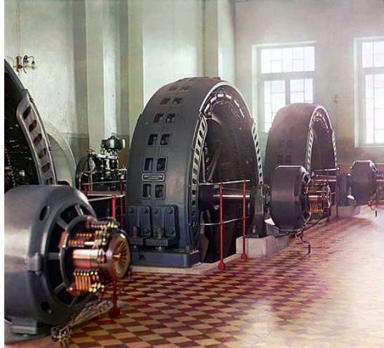
Рис. 5. Электрический генератор
